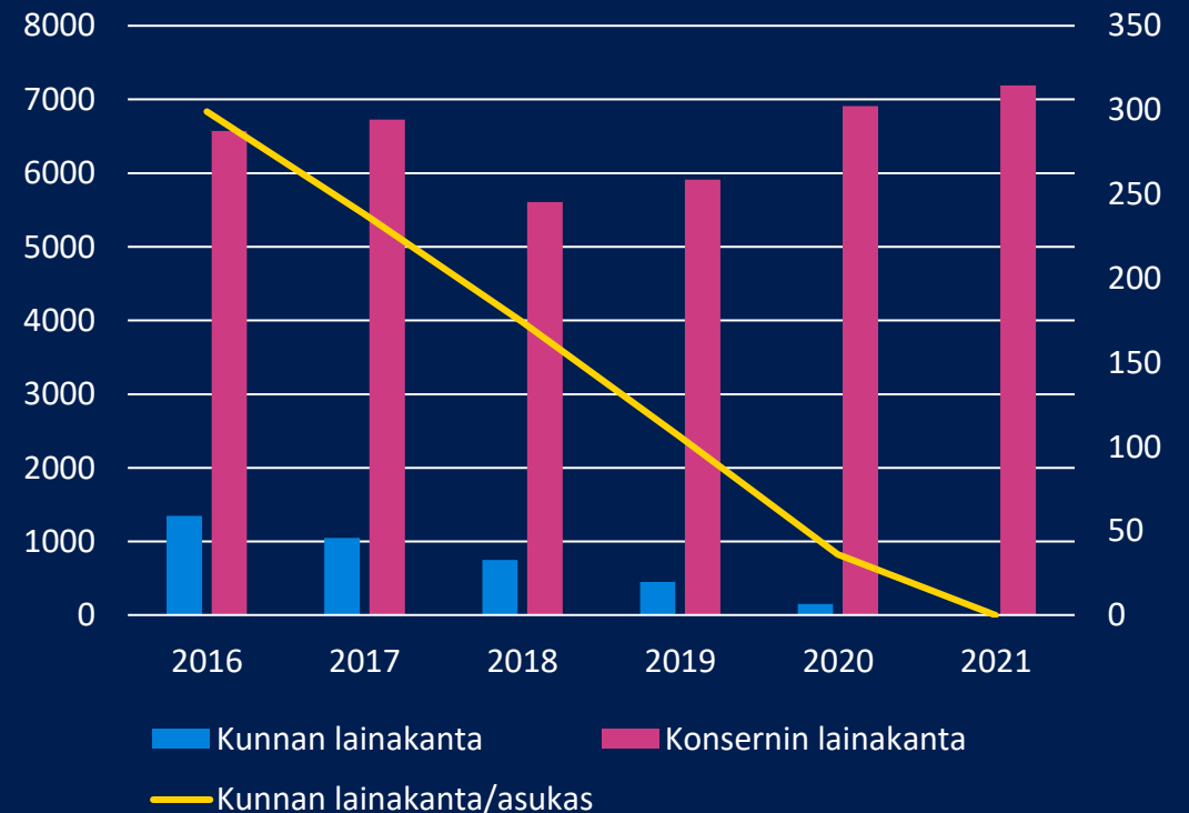
Kunnan ja konsernin lainakanta (1000 €) ja kunnan lainakanta/asukas €
