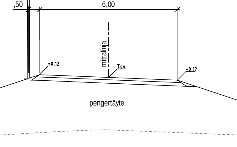
PENGER / POIKKILEIKKAUS 1:100 PLV 45-60 ja 147-210
