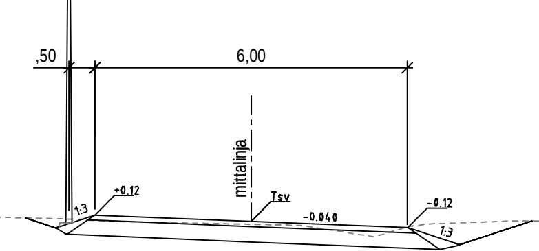
LEIKKAUS / POIKKILEIKKAUS 1:100 PLV 6-35 ja 220-270
