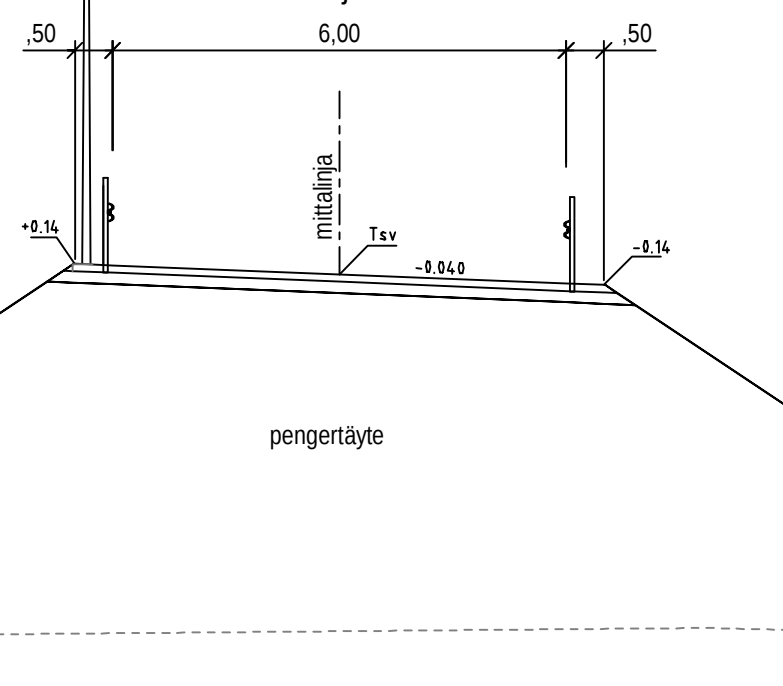
KAIDEPOIKKILEIKKAUS 1:100 PLV 70-90 ja 120-147
