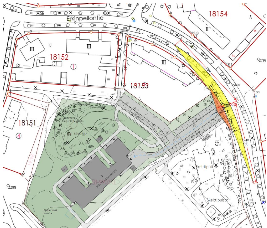
Kuva 9. Ajoliittymän näkemäalueet ja minimietäisyydet. Keltainen alue osoittaa sen alueen, jolle pysäköintialueelta poistuvan ajoneuvon kuljettajalla tulee olla esteetön näkyvyys.
