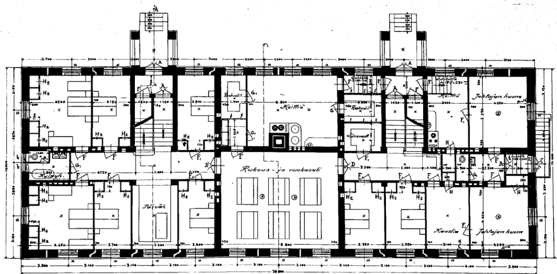
Ensimmäinen kerros
