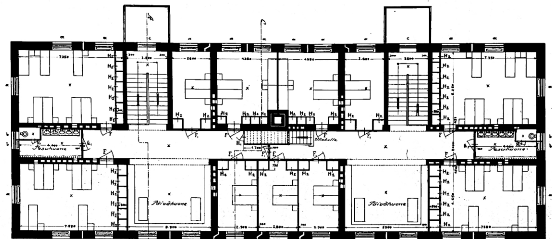
Toinen kerros
