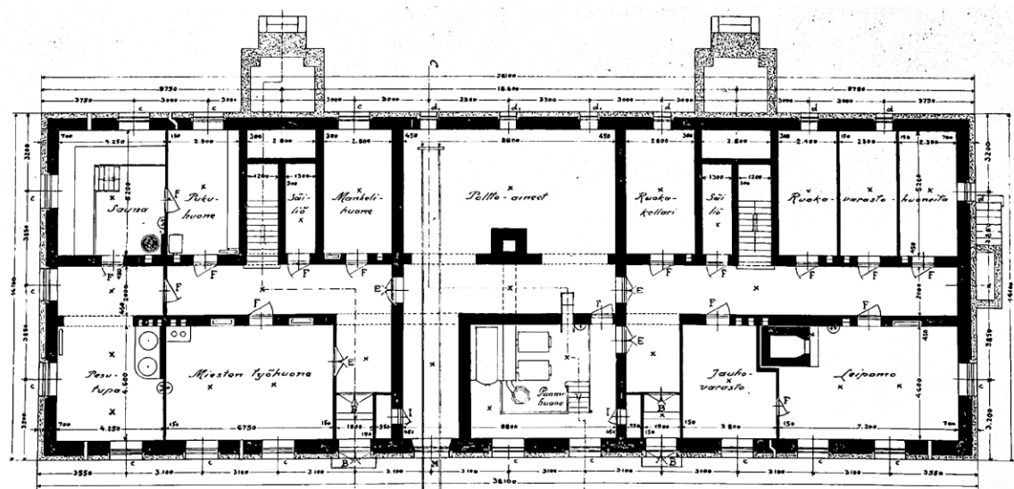
Kellarikerros.
