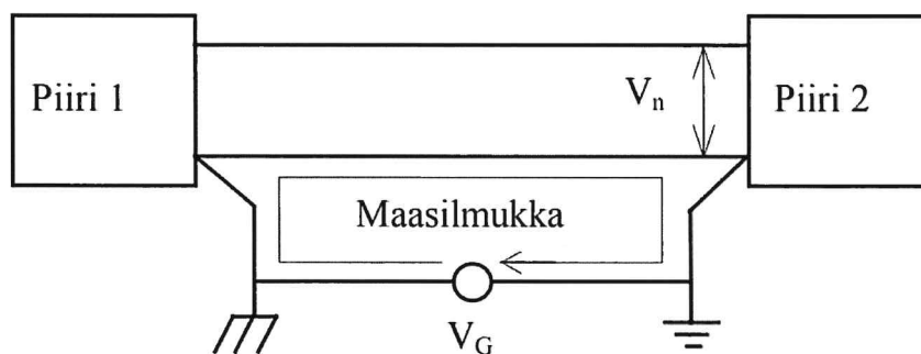
Kuva 8. Maasilmukan muodostuminen kahden piirin välille (ABB 2000)
