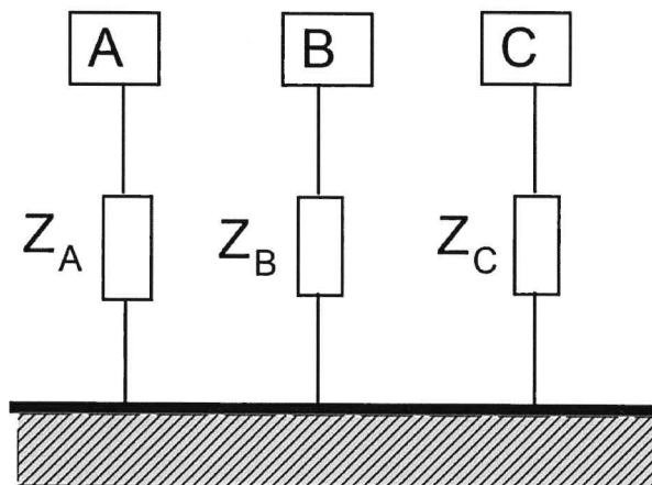
Kuva 7. Maadoituksen monipistekytkentä (ABB 2000)
