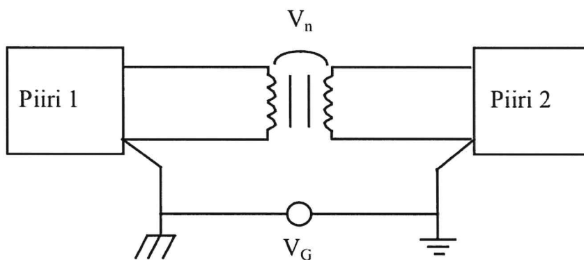
Kuva 9. Maasilmukan katkaiseminen muuntajaa käyttämällä (ABB 2000)
