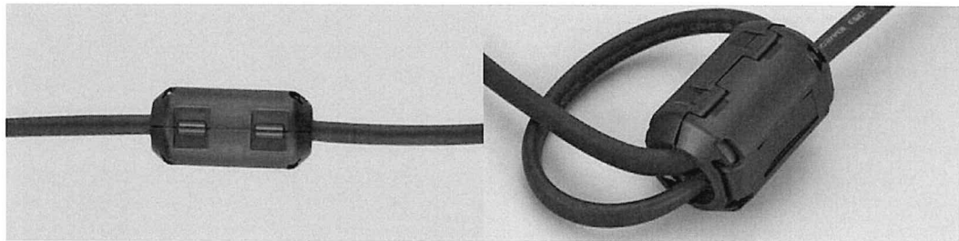
Kuva 11. Kaapelin ympärille asennettava ferriittirengas
