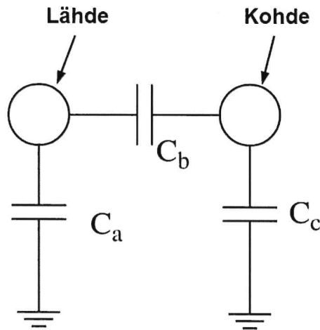
Kuva 2. Kapasitiivinen kytkeytyminen (Baker 2015, 62)
