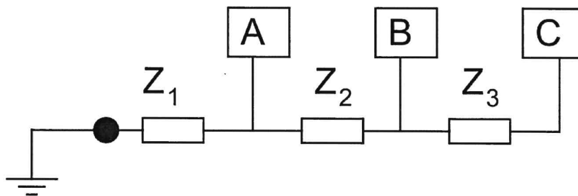
Kuva 5. Maadoituksen sarjakytkentä (ABB 2000)
