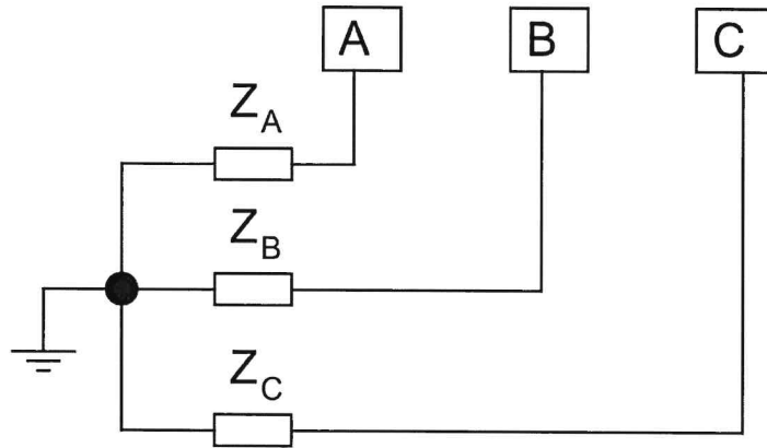
Kuva 6. Maadoituksen rinnankytkentä (ABB 2000)
