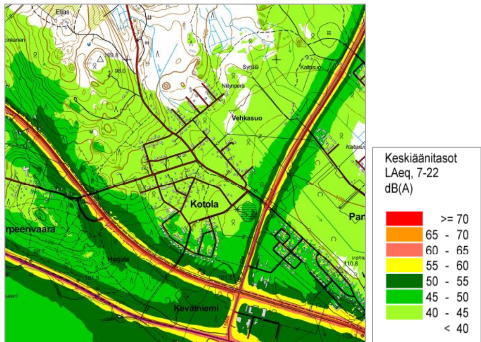
Kuva 23. Keskiäänitasot päivätaso uudessa nykytilanteessa, Biojalostamon asemakaavan meluselvitys (FCG, 6.2.2020).
