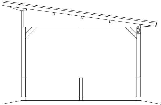
OIKEA SIVUSEINÄ
