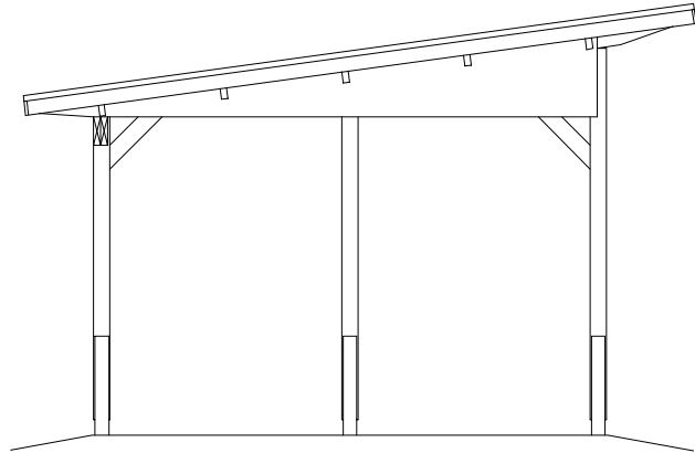
VASEN SIVUSEINÄ
