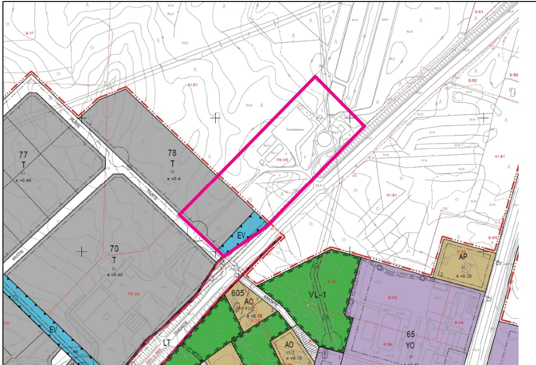
Kuva 4: Ote asemakaavakarttayhdistelmästä. Suunnittelualueen likimääräinen raja on esitetty pinkillä. Alueen pohjoisosa on kaavoittamatonta. Kartta: Tohmajärven kunta.
