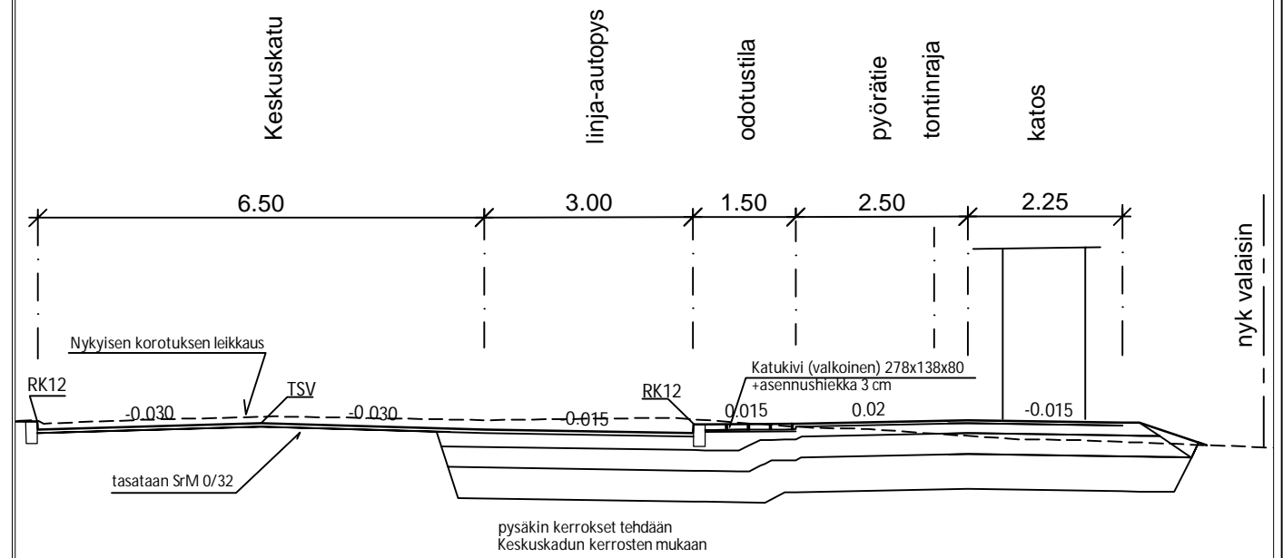
PÄÄLLYSRAKENNETAULUKKO LINJA-AUTOPYSÄKKI PYÖRÄTIE
