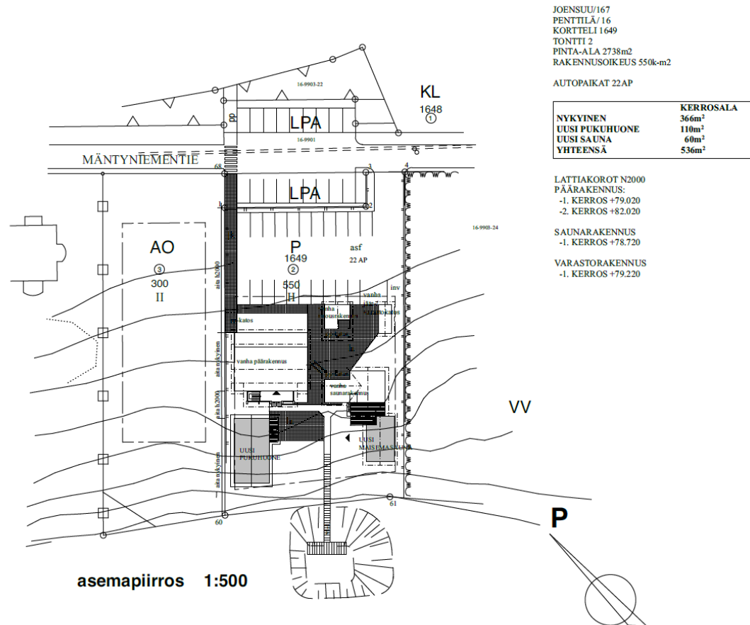
Kuva 26. Avantouintikeskuksen tontinkäyttösuunnitelma. Suuri osa rakennusoikeudesta käytetään pukutilojen ja toimistotilojen parantamiseen, sekä yhden uuden saunan rakentamiseen. Kokonaisrakennusoikeus on 550 k-m 2 .
