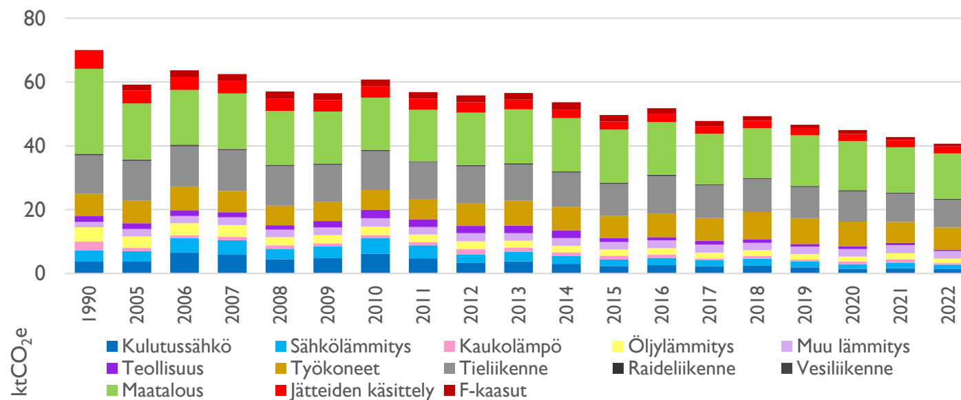
Kuvio 2: Juuan kasvihuonekaasupäästöjen kehitys päästösektoreittain 1990–2022
