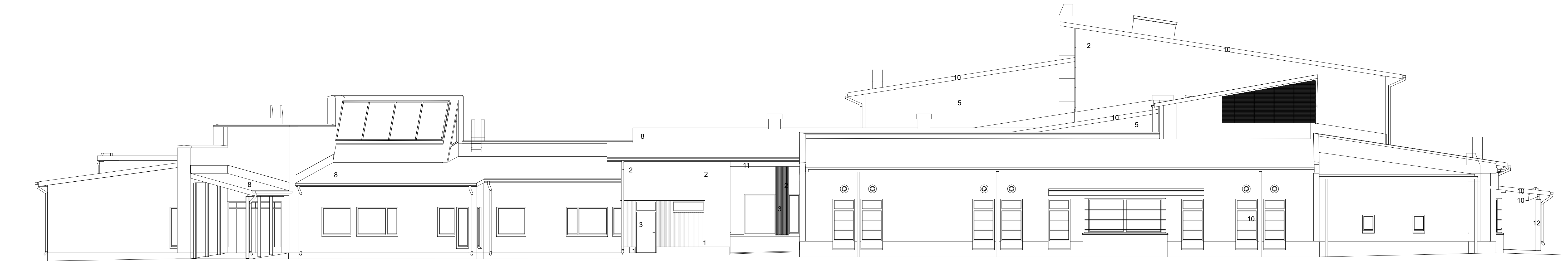
JULKISIVU ETELÄÄN
