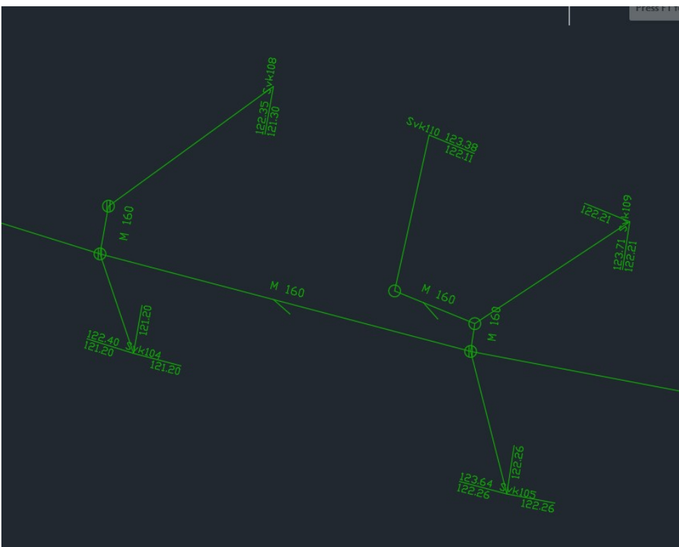
Kuva 5 Ote Valtimon verkostokartasta
