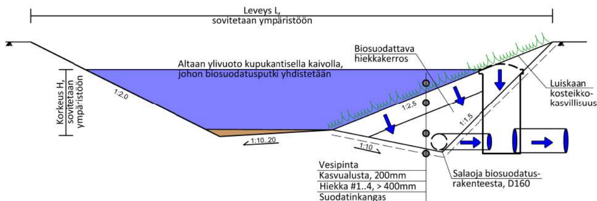
Kuva 10. Tyyppikuva biosuodatusrakenteesta, jossa suodatus tehdään luiskan kautta
