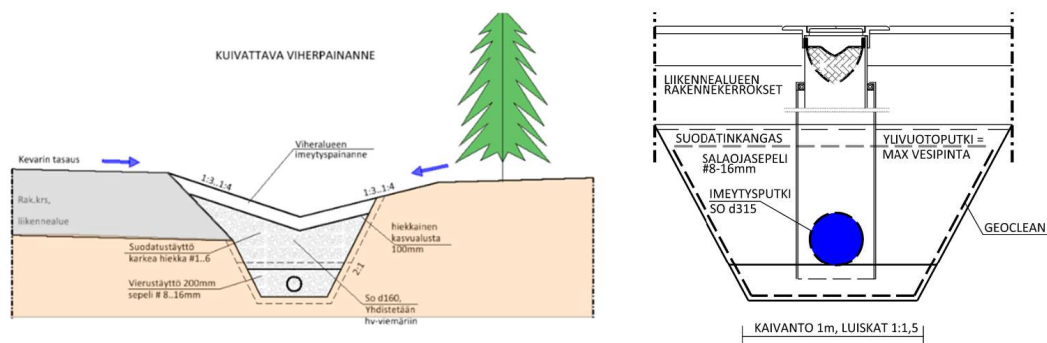
Kuva 9. Vasemmalla luonnonmukainen ja oikealla tekninen ratkaisu hulevesien suodattamiseen ja johtamiseen hidastettuna vastaanottavaan järjestelmään (kuvat Watec Consulting).
